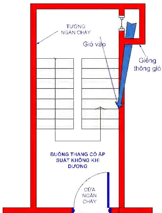
a) Buồng thang bộ không nhiễm khói loại N2
