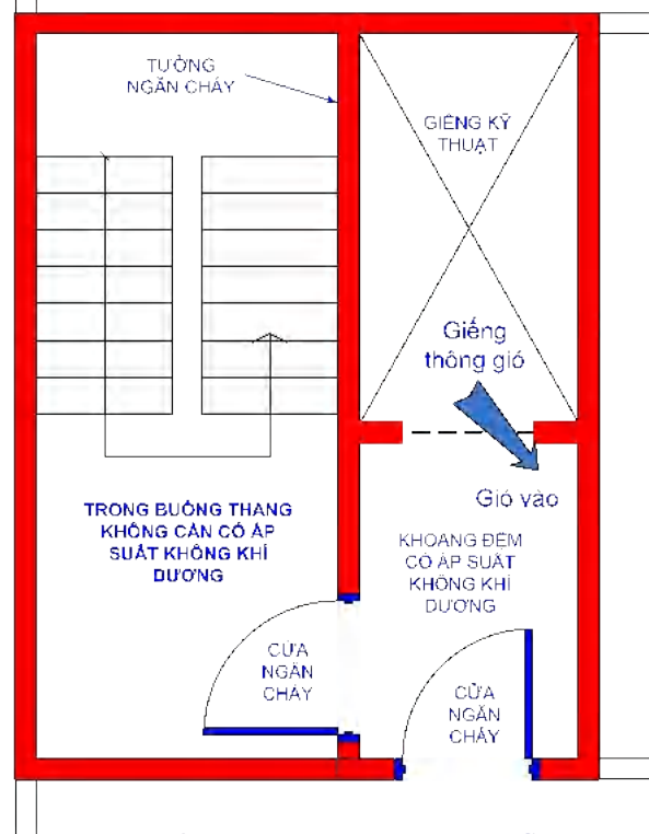
b) Buồng thang bộ không nhiễm khói loại N3
