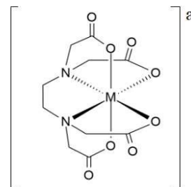
Phức chất của cation kim loại \text{M}^{n+} với phối tử EDTA
