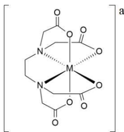
Phức chất của cation kim loại \text{M}^{n+} với phối tử EDTA
