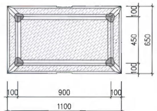
MẶT BẰNG LỒNG KÍNH
