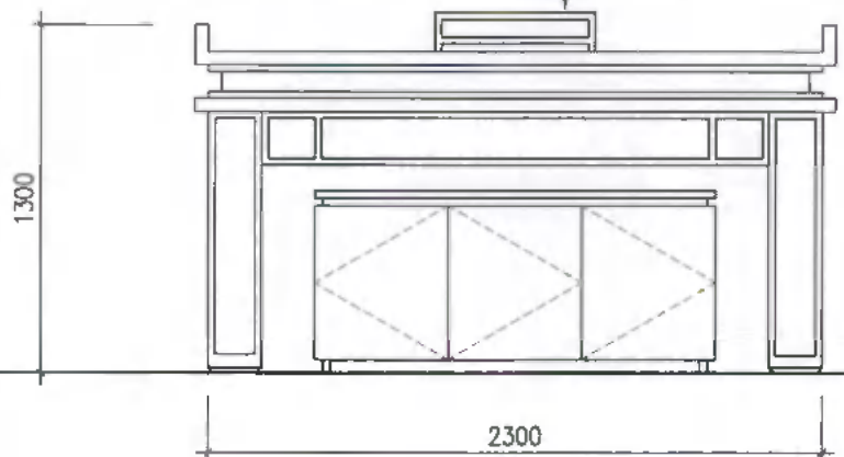
MẶT ĐỨNG CHÍNH
