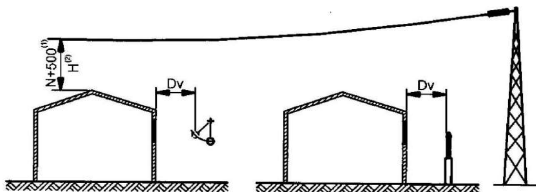
Hình 3.6: Khoảng cách tiếp cận nhỏ nhất đến khung vận chuyển
