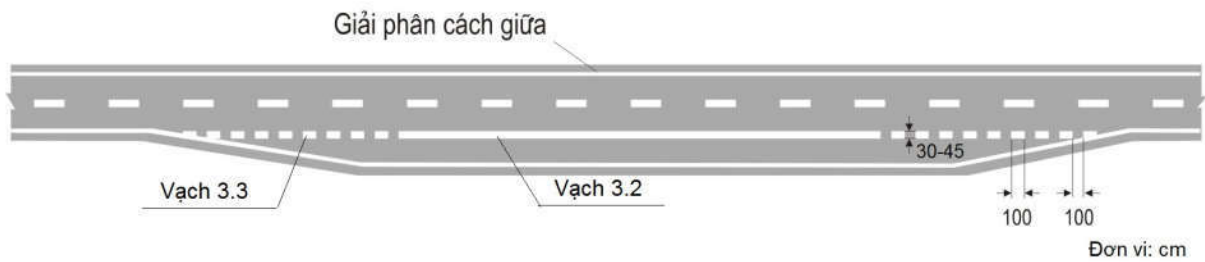
Hình G.18 - Bố trí vạch ở điểm dừng xe kiểu bến cảng không có đảo sơn phân làn
