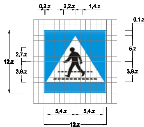
Biển số I.423b : Vị trí người đi bộ sang ngang
