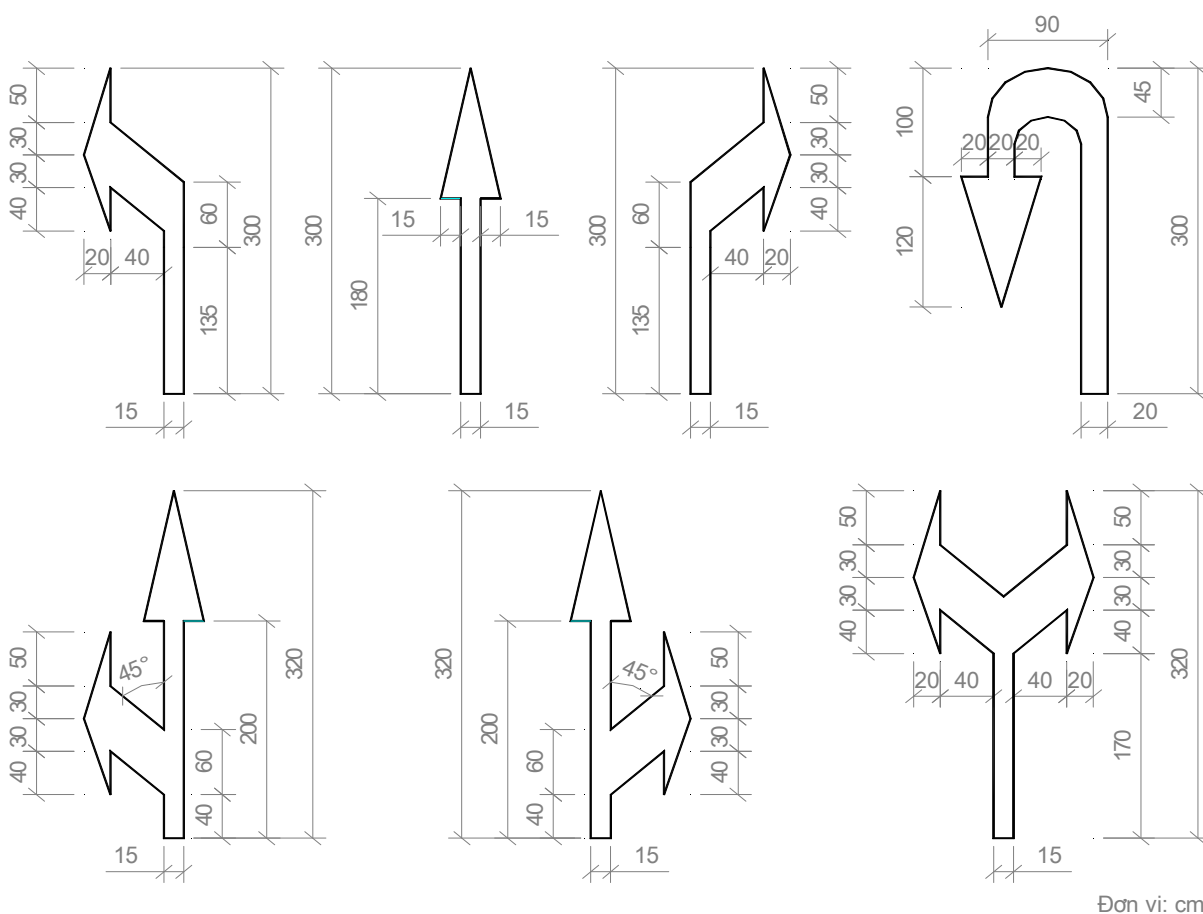
Hình G.73 - Kích thước mũi tên chỉ đường áp dụng cho đường có tốc độ xe chạy thấp
