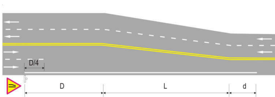
Hình G.22 - Bố trí vạch sơn khu vực chuyển tiếp giữa đường 4 làn xe và đường 3 làn xe
