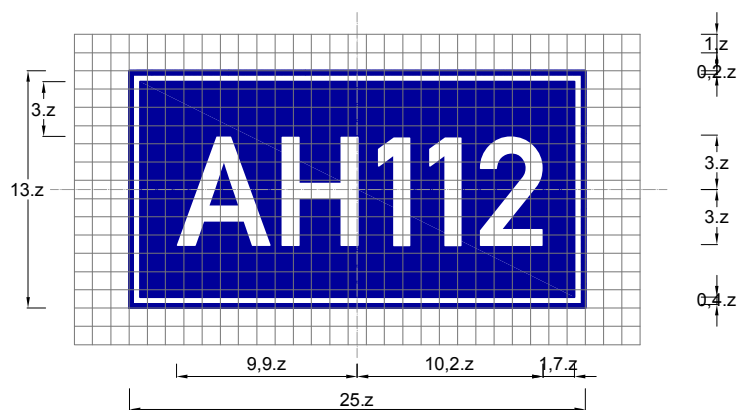
Biển số I.449 : Biển tên đường
