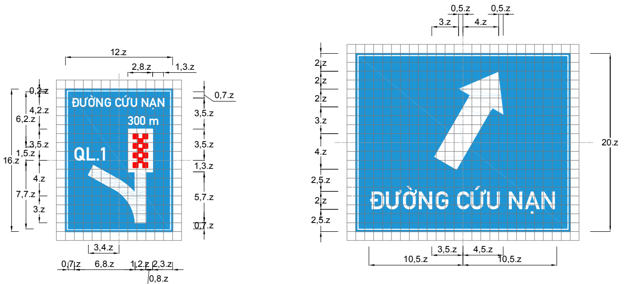
Biển số I.448 : Làn đường cứu nạn hay làn thoát xe khẩn cấp
