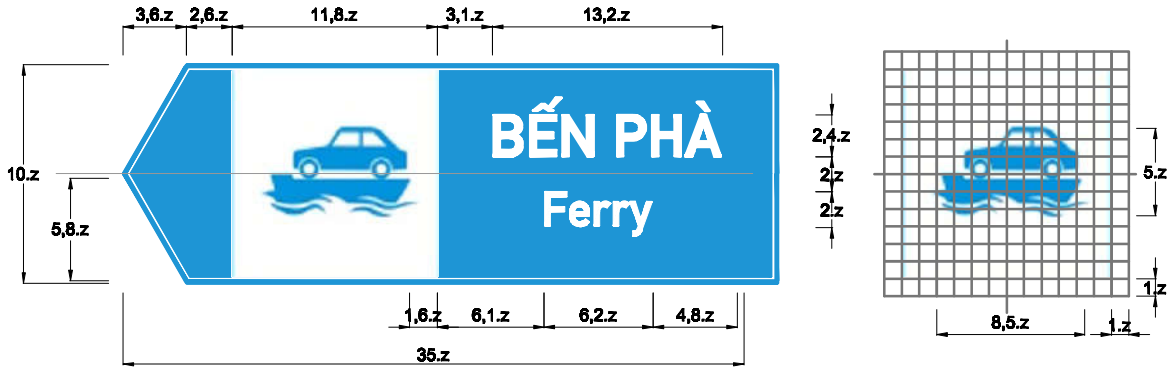
Biển số I.44j : Biển báo chỉ dẫn địa điểm
