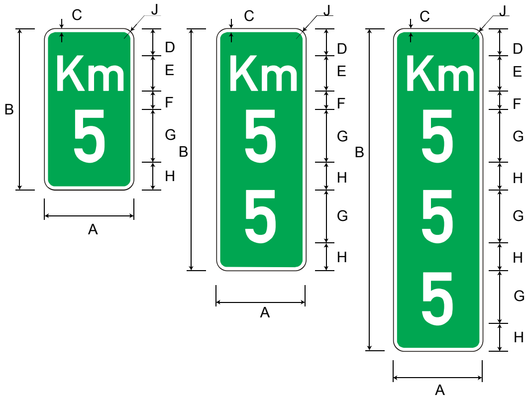
a) Loại một chữ số lý trình b) Loại hai chữ số lý trình c) Loại ba chữ số lý trình
