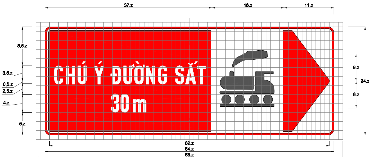
Biển số S.510b : Chú ý đường sắt
