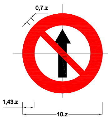
Biển số P.136: Cấm đi thẳng
