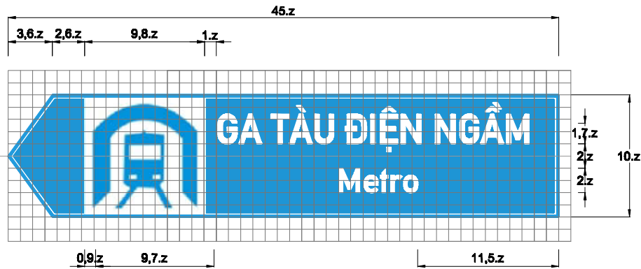
Biển số I.44k : Biển báo chỉ dẫn địa điểm
