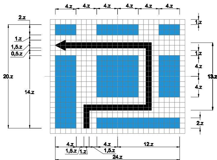
Biển số I.419a : Chỉ dẫn địa giới 24z (Thay đổi tùy theo số lượng chữ)
