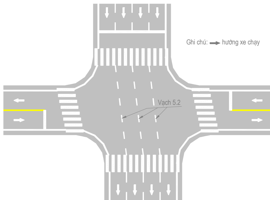
Hình G.41 - Minh họa bố trí vạch 5.2
