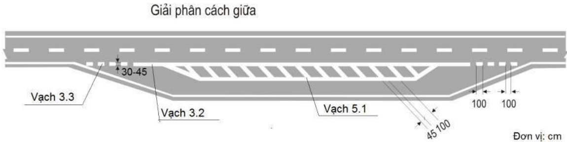
Hình G.19 - Bố trí vạch ở điểm dừng xe kiểu bến cảng, trường hợp sử dụng vạch 5.1
